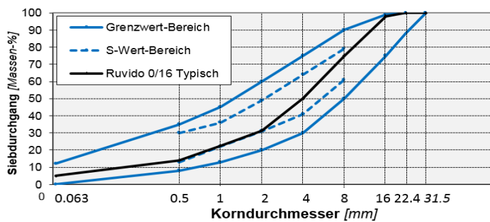
Typische Korngrößenverteilung von Ruvido 0/16 (EOS-Granulat)
