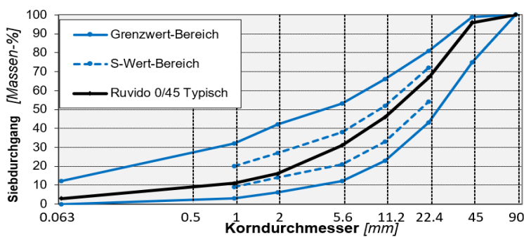
Typische Korngrößenverteilung von Ruvido 0/45S (EOS-Granulat)
